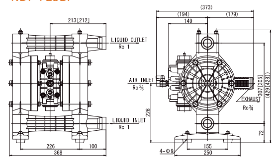
NDP-P25BP
