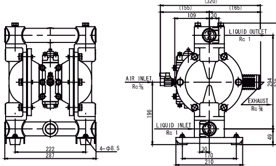
NDP-25BA
